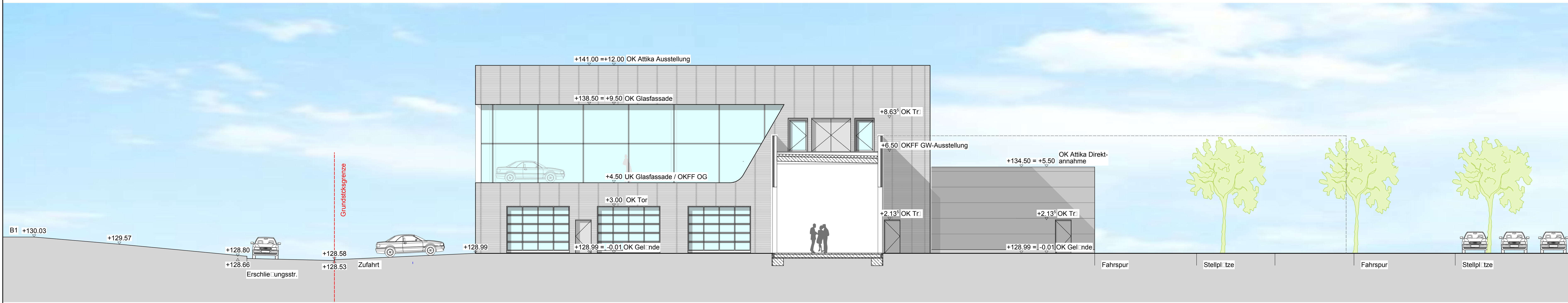
SNITT B-B M 1:100
