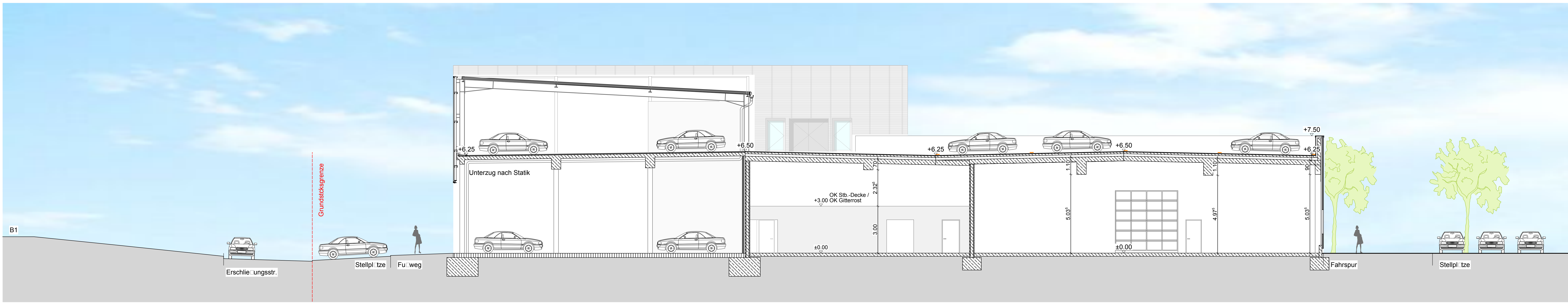
SNITT C-C M 1:100
