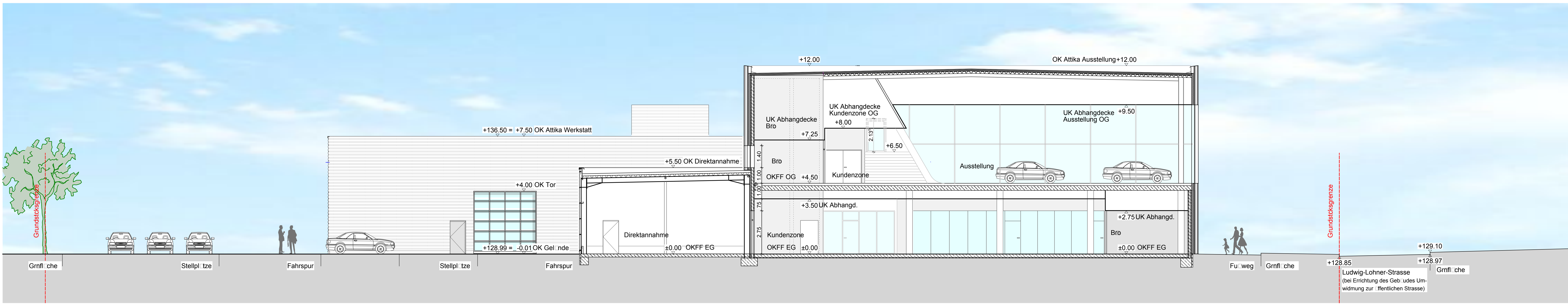
SNITT E-E M 1:100
