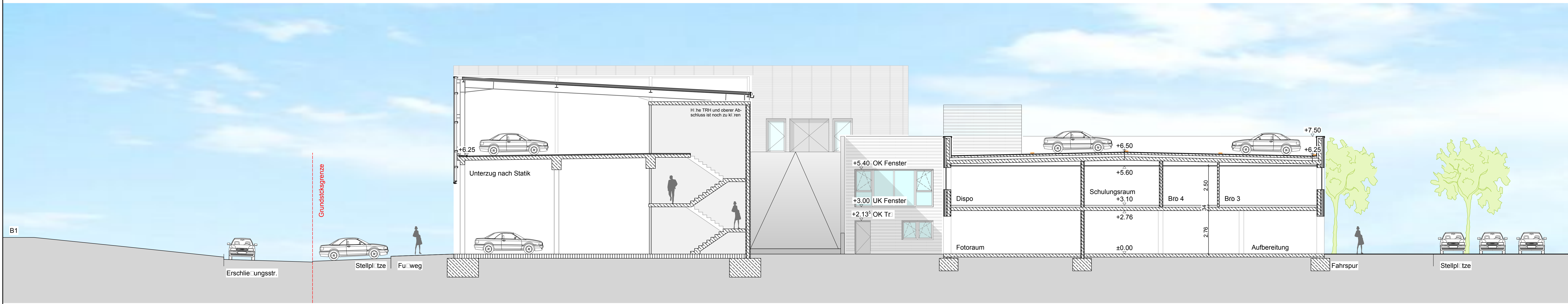
SNITT D-D M 1:100
